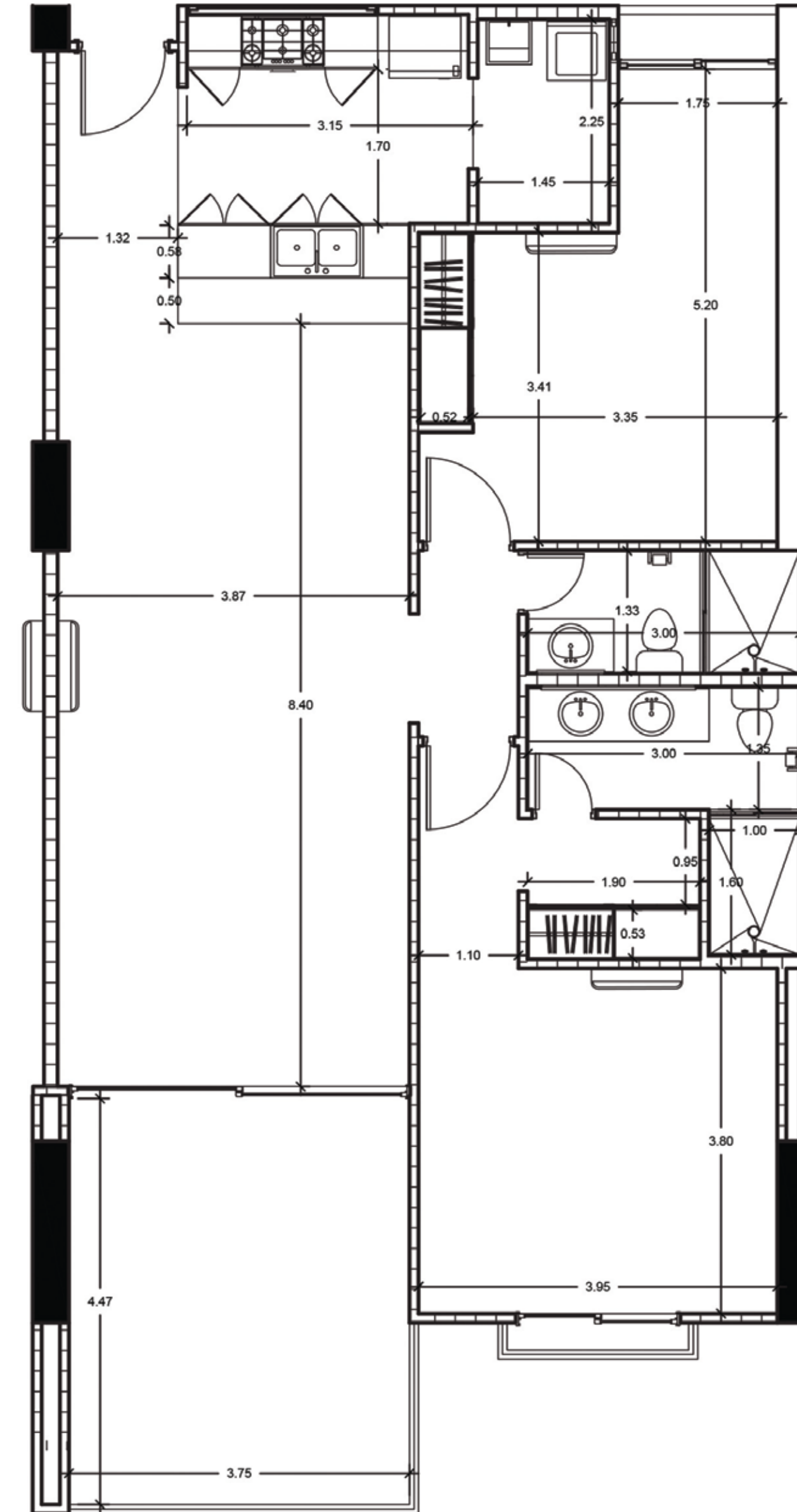
Planta arquitectónica Modelo B - 125 mts2
