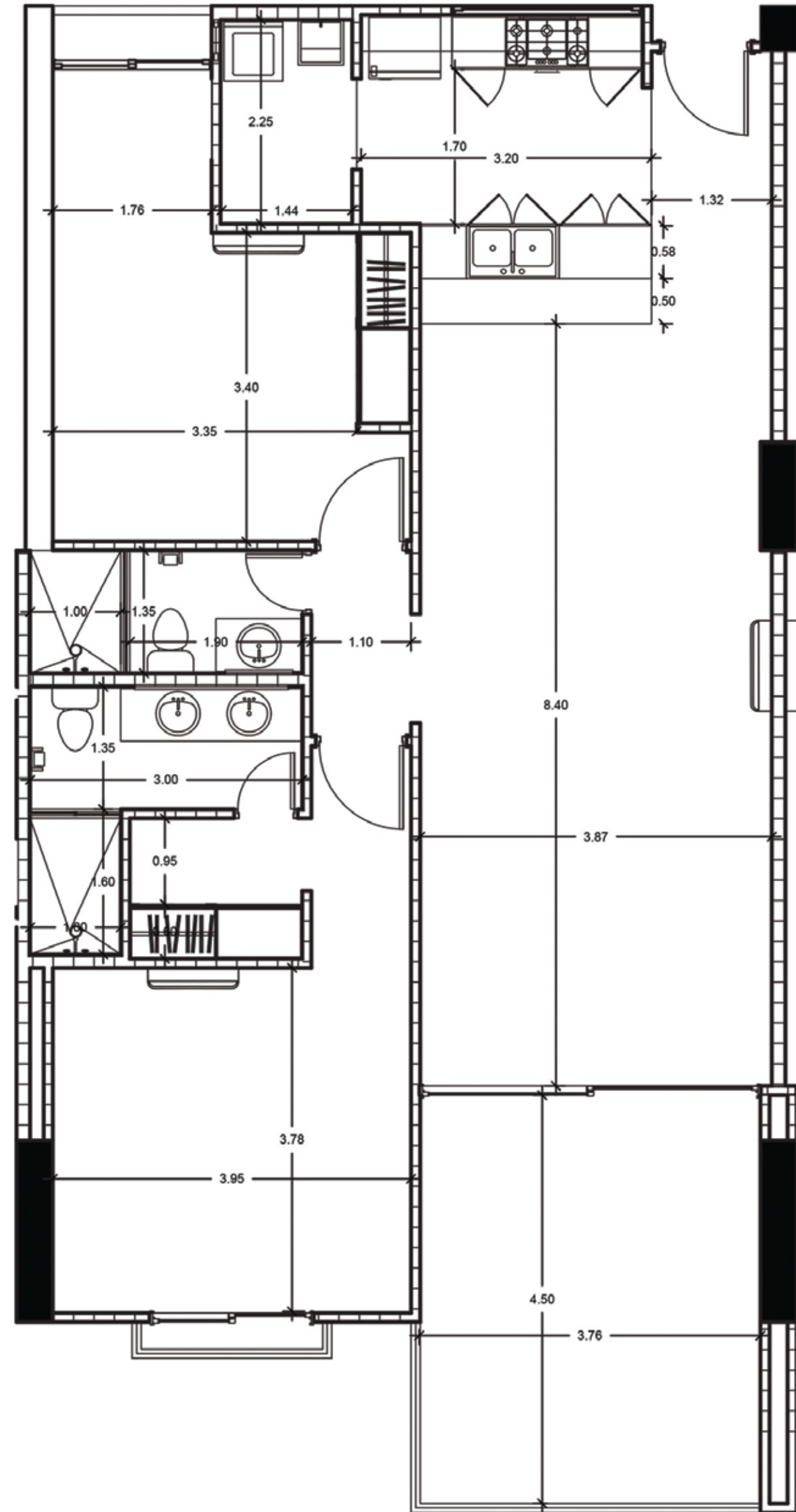
Planta arquitectónica Modelo D - 125 mts2
