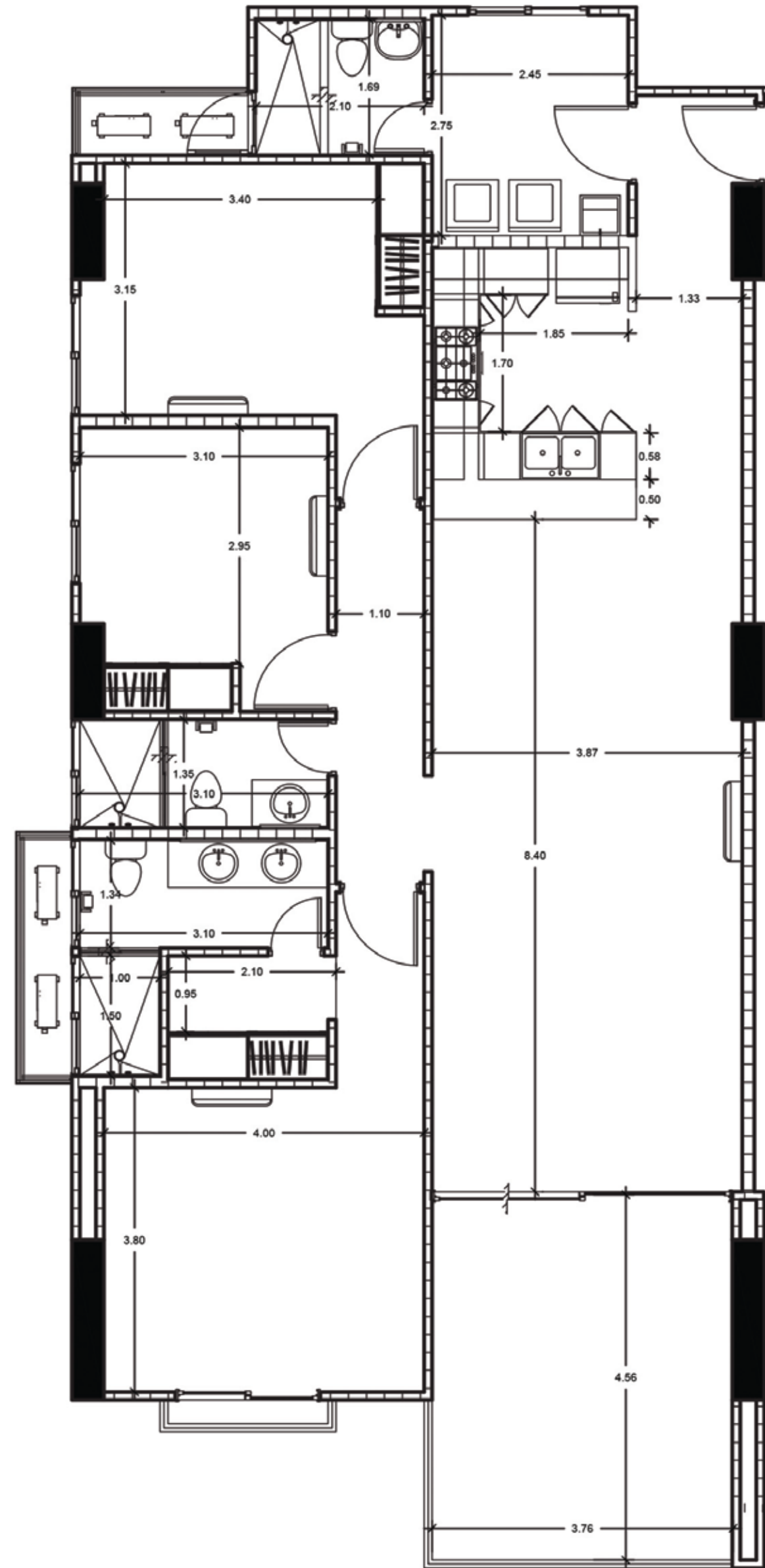
Planta arquitectónica Modelo A - 152 mts2
